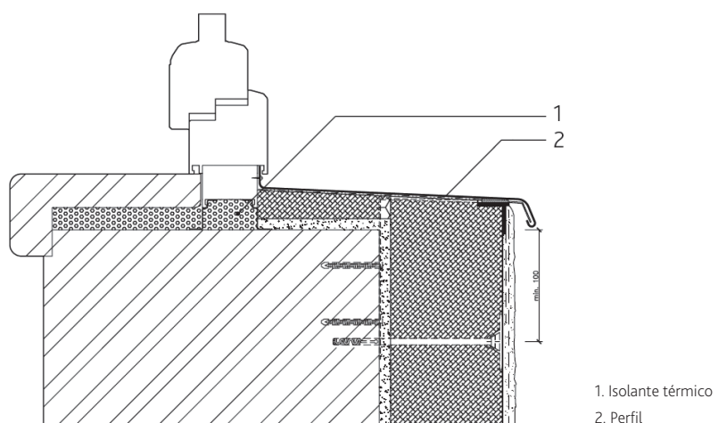
Corte vertical de uma janela
