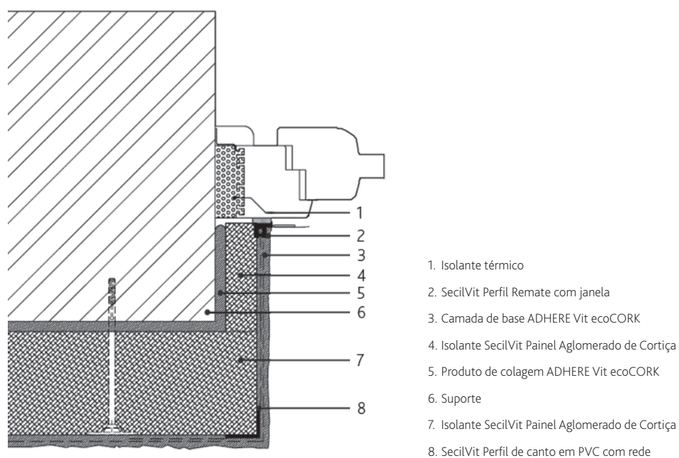
Corte horizontal de uma janela
