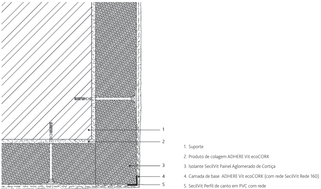
Corte horizontal de uma esquina com perfil de canto
