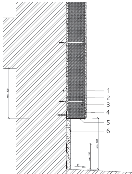
Corte vertical do arranque do sistema
